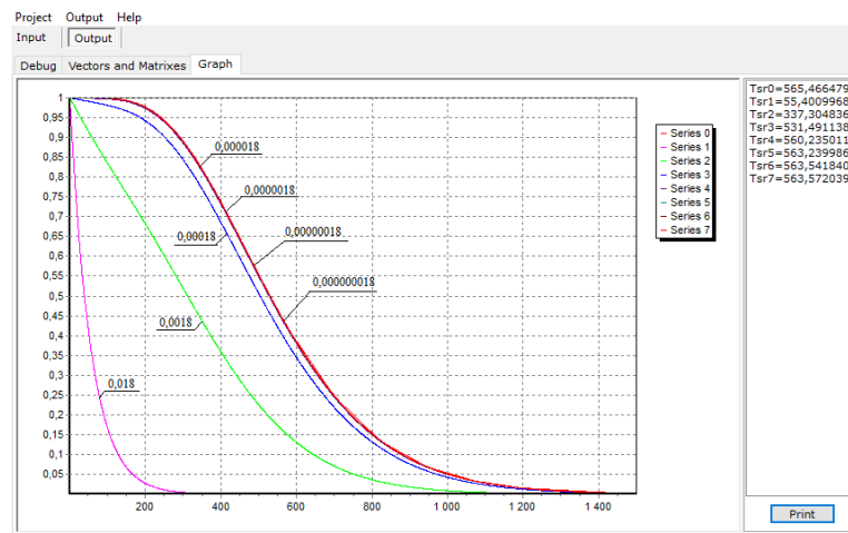
Рис. 4. Залежність ймовірності безвідмовної роботи системи передавання даних від часу експлуатації при різних значеннях інтенсивності відмов комутатора (від 1,8 \cdot 10^{-2} до 1,8 \cdot 10^{-8} год -1 )
