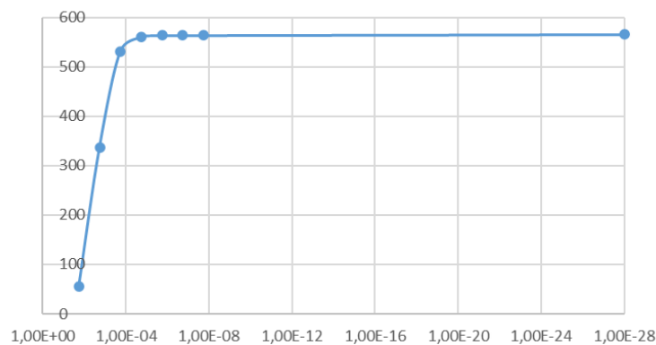
Рис. 5 Залежність середнього часу роботи до відмови (МТТФ) системи передавання даних від інтенсивності відмов комутатора
