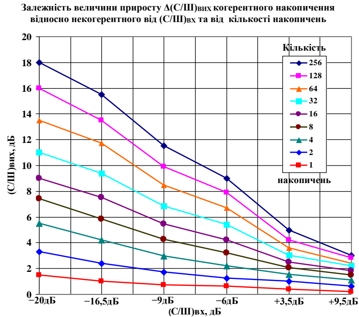
Рис.4. Залежність приросту вихідного відношення \Delta(C/Ш)_{вих} когерентного накопичення відносно некогерентного при різних значеннях вхідного відношення (C/Ш)_{вх} та різних кількостях накопичень сигналів
