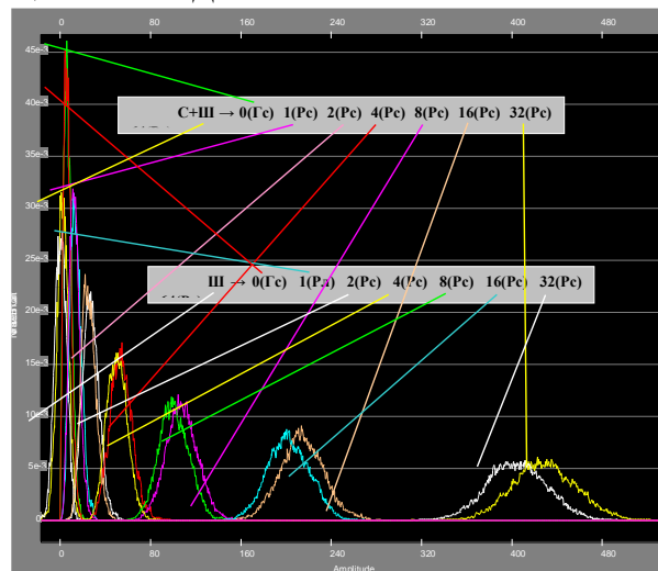
Рис.6. Процес трансформації густин ймовірностей вихідного сигналу або шуму для різних кількостей (1, 2, 4, 8, 16, 32, 64) накопичень при конкретному значенні вхідного відношення (C/Ш)_{ВХ} = -9,2 дБ (некогерентний режим)
