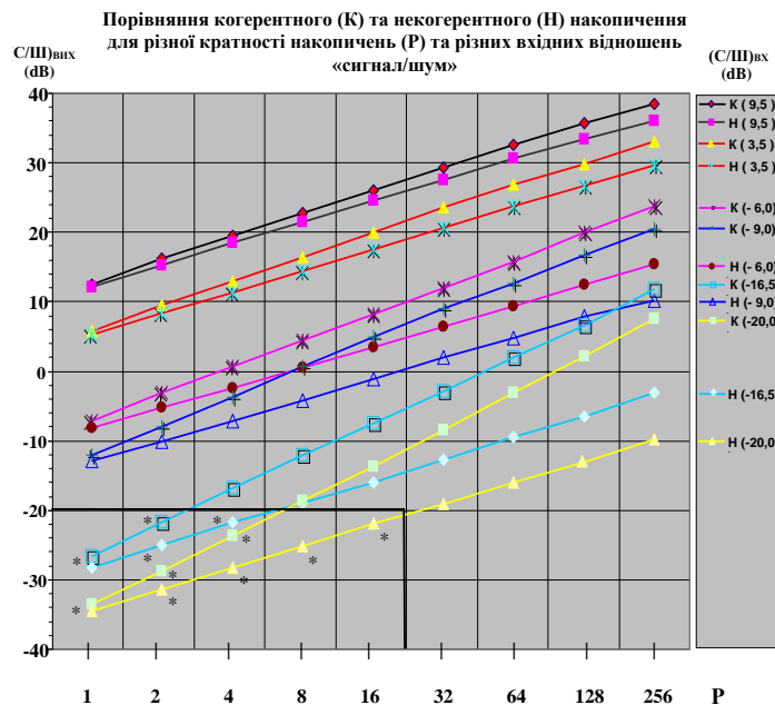
Рис.3. Залежність вихідного відношення (C/Ш)_{ВІХ} від деяких різних значень вхідного відношення (C/Ш)_{ВХ} при різних кількостях накопичень сигналів
