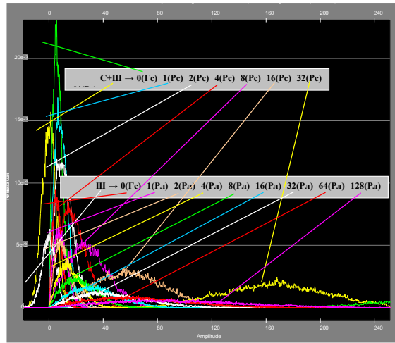
Рис.5. Процес трансформації густин ймовірностей вихідного сигналу або шуму для різних кількостей (1, 2, 4, 8, 16, 32, 64) накопичень при конкретному значенні вхідного відношення (C/Ш)_{ВХ} = -9,2 дБ (когерентний режим)
