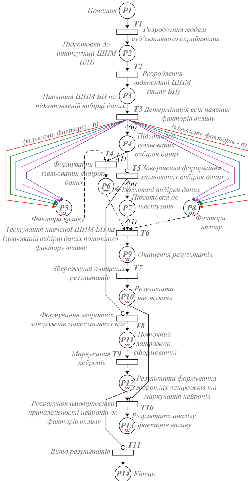
Рис. 3. Модель аналізу факторів впливу автоматизації підтримки програмних комплексів на базі кольорових мережі Петрі. (Продовження)
