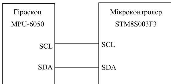
Рис.3. Схема під'єднання гіроскопа MPU-6050 до мікроконтролера STM8S003F3 з використанням інтерфейсу I2C
