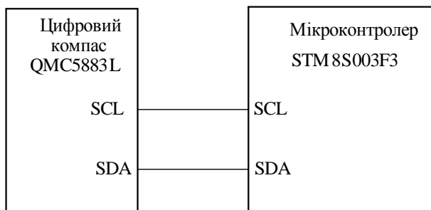
Рис. 4. Схема під'єднання цифрового компаса HMC5883/QMC5883L до мікроконтролера STM8S003F3 з використанням інтерфейсу I2C
