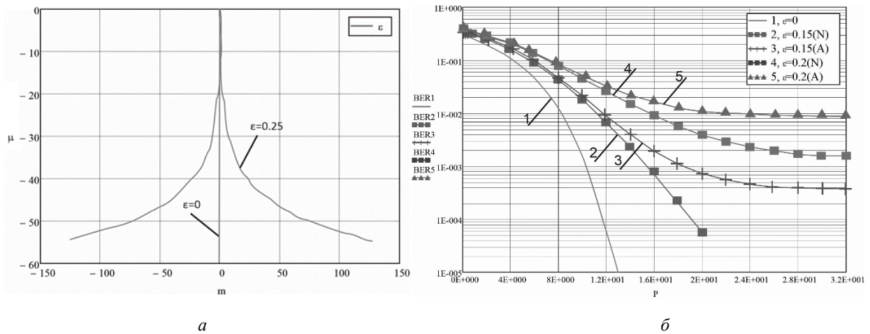
Рис. 3. Залежності для оцінювання частотних спотворень: а – коефіцієнтів M_{k3} - \mu_m (у дБ) у випадку коли зміщення частоти \varepsilon дорівнює 0 та 0,25; криві заводостійкості оптичної-OFDM системи у випадку зсуву частоти (формувалось 256 піднесучих типу ФМ-4): \varepsilon – нормоване значення зміщення частоти відносно до рознесення піднесучих
