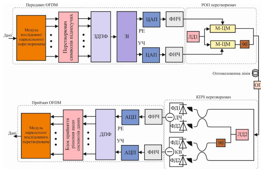
Рис. 1. Функціональна схема КО-OFDM каналу з подвійною конвертацією сигналів: ЗДПФ – блок зворотного перетворення Фур’є; ЗІ – блок утворення захисного інтервалу; ЦАП/АЦП – блоки цифро-аналогового та аналого-цифрового перетворення; ФНЧ – фільтри низьких частот; ЛД- лазерний діод; М-ЦМ – модулятор Маха-Цендера [17, 18]; 90° – фазообертач; ФД – фотодіод; ДЧ/КВ – дійсна та квадратурна складова сигналу; РЕ/УЧ – реальна та уявна частина сигналу
