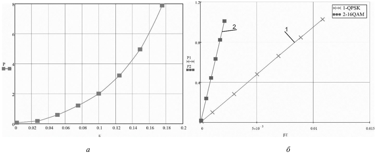
Рис. 4. Залежності для оцінювання фазо-частотних спотворень: а – графік який показує результат погіршення С/Ш (P) як залежність від функції зміщення частоти ( \epsilon ) для оптичної-OFDM (ФМ-4 (QPSK); 256-піднесучих); б – графік зміни відношення С/Ш (P) залежно від ширини лінії в оптичних-OFDM для випадку застосування в каналі сигналів типу ФМ-4 та КАМ-16 (16QAM)
