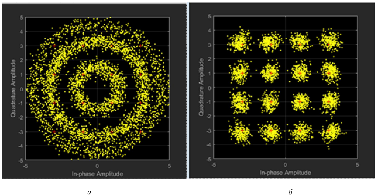
Рис. 5. Графіки (сузір'я) для оцінювання впливу дисперсії на сигнали багатопозиційної маніпуляції типу КАМ-16: а – після каналу під дією дисперсії; б – відновлений сигнал після компенсації впливу дисперсії
