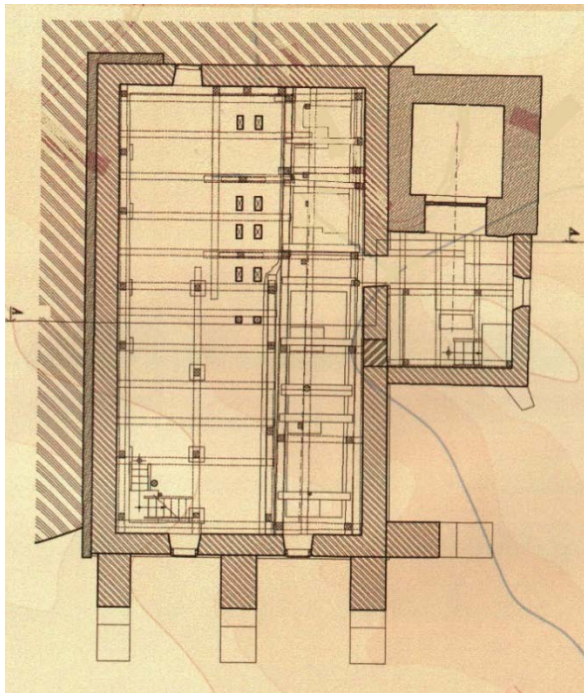
Рис. 14. план цокольного поверху млина у Васючині. Опрацювання О. та І. Бокало (Бокало, 2006).
