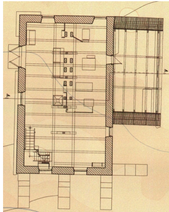
Рис. 15. План 1-го поверху млина у Васючині. Опрацювання О. та І. Бокало (Бокало, 2006).
