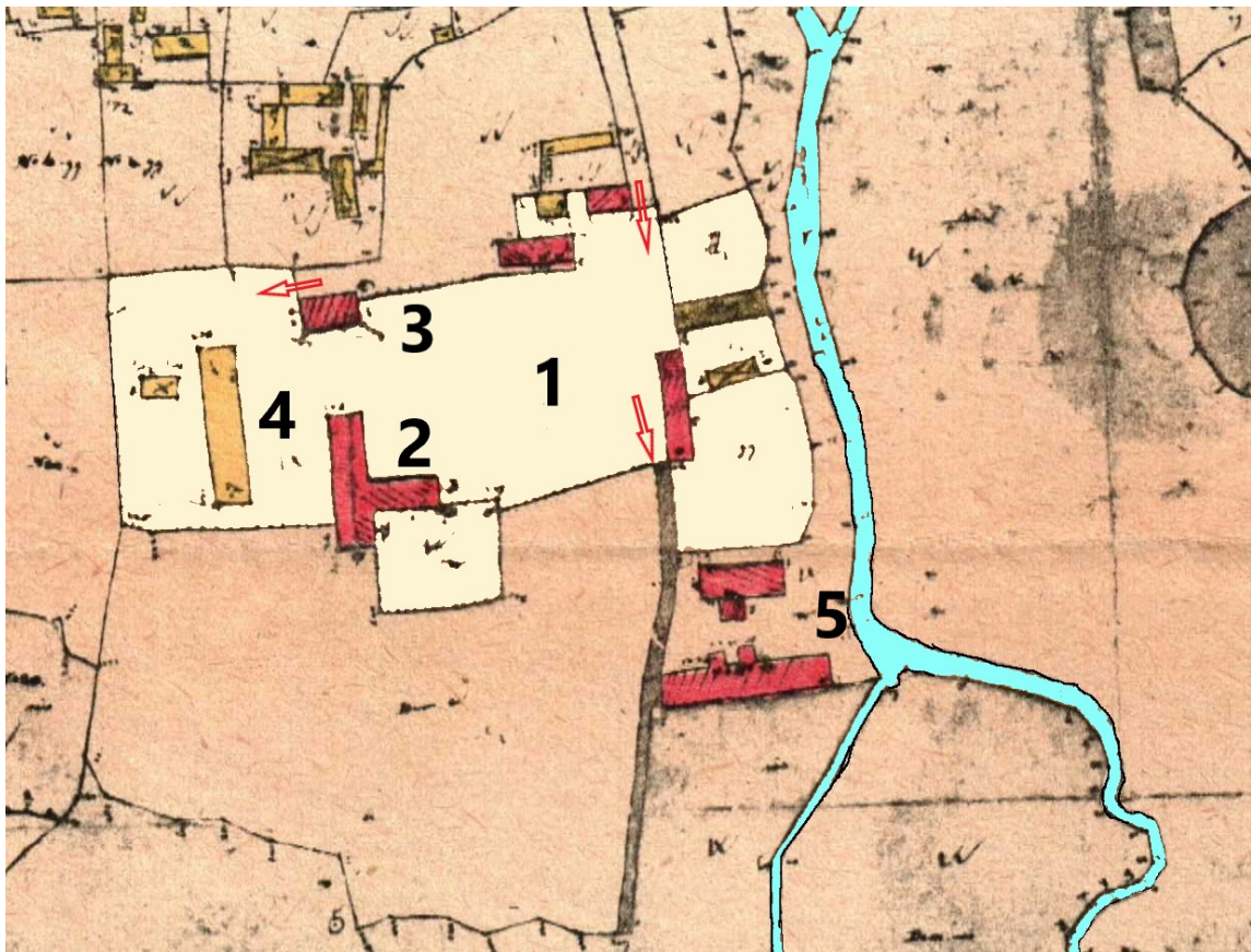
Рис. 6. Територія колишнього замку у Васючині на брульйон-плані поселення з 1846 р. (ЦДІА, 1846). Умовні позначення: червоним кольором позначено муровані будівлі, жовтим кольором – дерев'яні; цифрами позначено: 1 – двір, 2 – палацова будівля, 3 – кухня та пекарня, 4 – шпихлір та комори, 5 – будівлі алебастрової майстерні. Навколо двору (1) розміщені також інші господарські будівлі – возівня, стайні, житло прислуги. Опрацювання – М.Бевз.
