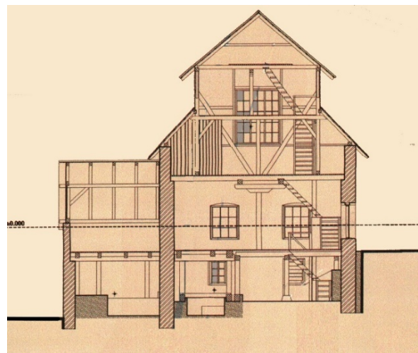
Рис. 17. Поперечний перетин по споруді млина у Васючині. Опрацювання О. та І. Бокало (Бокало, 2006).
