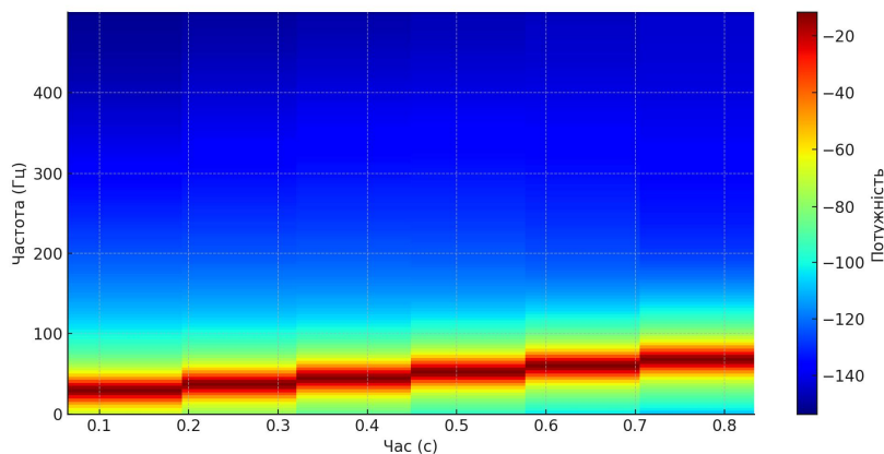
Рис. 14. Спектрограма сигналу з ЧРС
