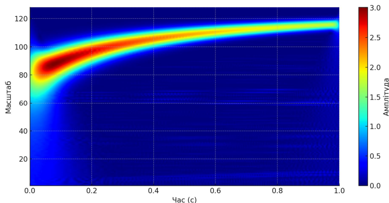
Рис. 16. Чирп-вейвлет сигналу з ЧРС
