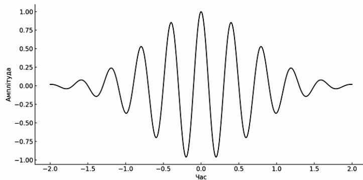
Рис. 1. Вейвлет Морле
