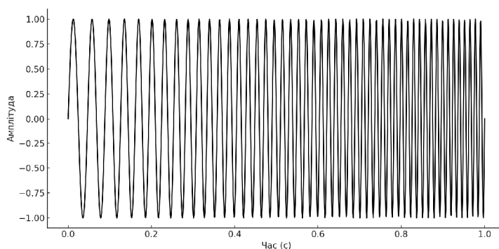
Рис. 10. Досліджуваний сигнал із ЧРС
