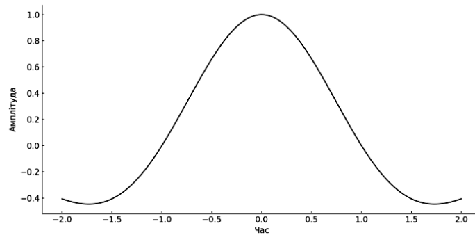
Рис. 2. Вейвлет “Мексиканський капелюх”
