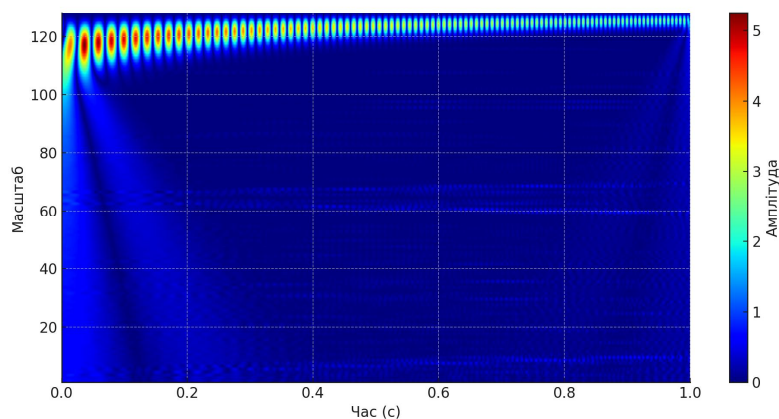
Рис. 15. Вейвлет “Мексиканський капелюх” сигналу з ЧРС
