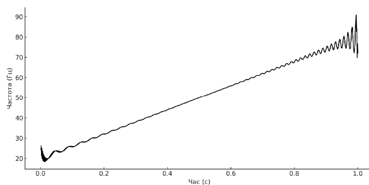
Рис. 12. Миттєва частота сигналу з ЧРС
