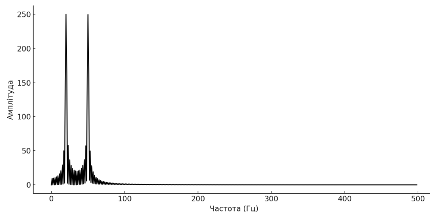
Рис. 4. ШПФ сигналу ППРЧ
