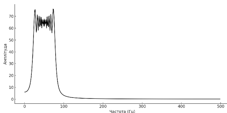
Рис. 11. ШПФ сигналу із ЧРС
