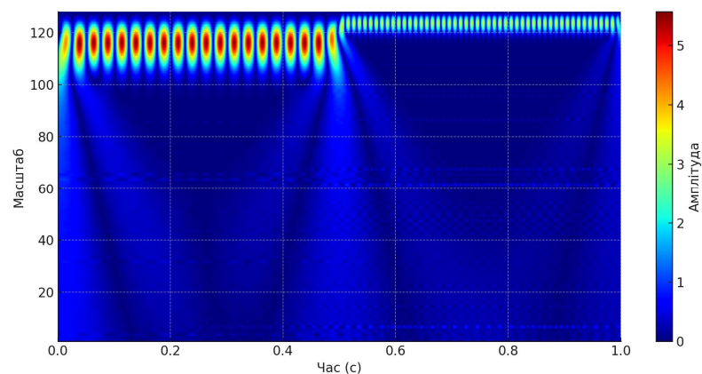
Рис. 8. Вейвлет “Мексиканський капелюх” сигналу ППРЧ
