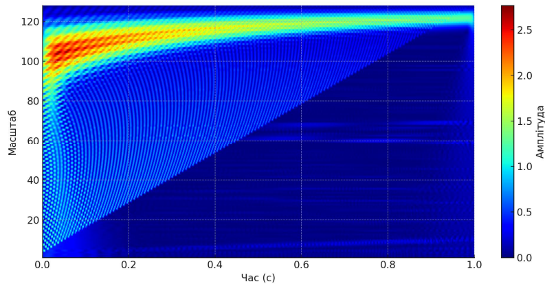
Рис. 13. Вейвлет Морле сигналу з ЧРС
