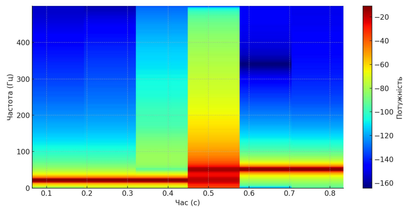
Рис. 7. Спектрограма сигналу ППРЧ
