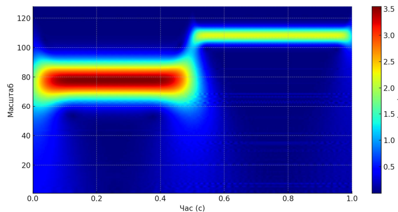
Рис. 9. Чирп-вейвлет сигналу ППРЧ
