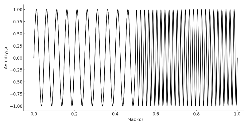
Рис. 3. Досліджуваний сигнал із ППРЧ
