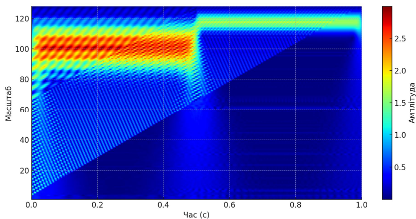
Рис. 6. Вейвлет Морле для сигналу ППРЧ
