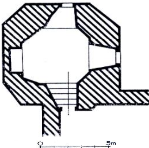
Рис. 5. Обмірне креслення третього ярусу вежі Поворозників з праці Я. Вітвіцького (Witwicki, 1971)
