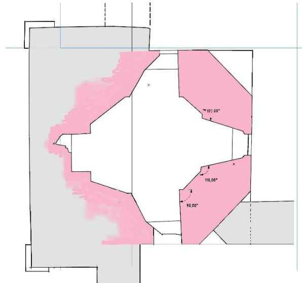
Рис. 6. Обмірне креслення третього ярусу вежі Поворозників. Рожевим кольором позначено цегляне мурування, сірим – кам'яне (кафедра архітектури та реставрації, кресленик М. Каплінська, М. Бевз, 2025)
