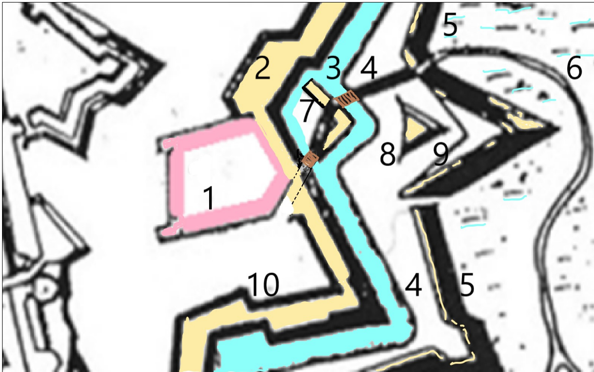
Рис. 6. Фрагмент плану укріплень Львова Яна Беренса (позначення кольором елементів фортифікації та експлікація додана авторами). 1 – монастир Кармелітів Черевичкових; 2 – основний внутрішній вал оборонної лінії Беренса оскарпований із зовнішньої сторони муром; 3 – фосою з водою; 4 – гласис; 5 – зовнішній земляний вал лінії Беренса; 6 – дорога візду до міста; 7 – трикутний равелін оточений фосою з мостами перед візною брамою у внутрішньому валі; 8 – трикутний редан перед равеліном на зовнішньому контргардному валі; 9 – додатковий вал перед реданом на трикутному бастіоні контргардного зовнішнього валу; 10 – великий наріжний бастіон з казематами у місці нинішніх вулиць Фредра та проспекту Т.Шевченка. Опрацювання В.Бевз.
